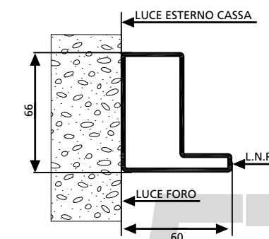
Telaio senza aletta
