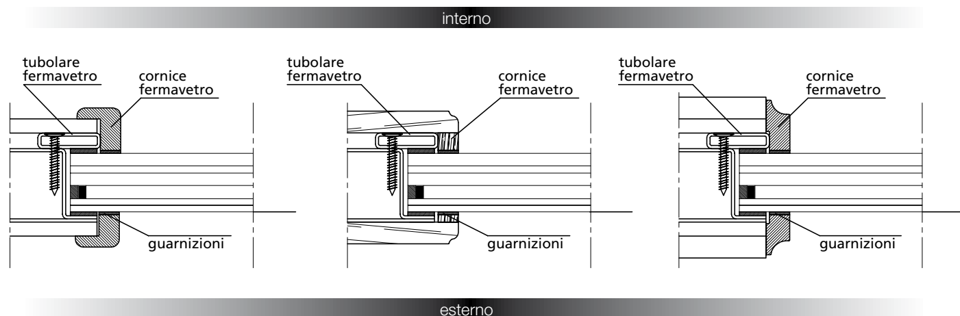
Sezione pannelli piani
