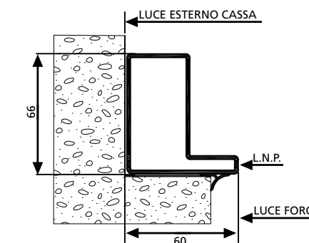
Telaio senza aletta
