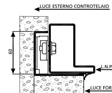
Telaio senza aletta su controtelaio
